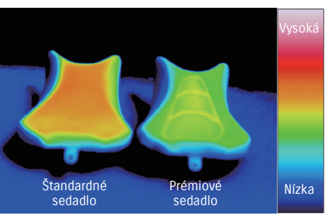
Termografické porovnanie povrchových teplôt
